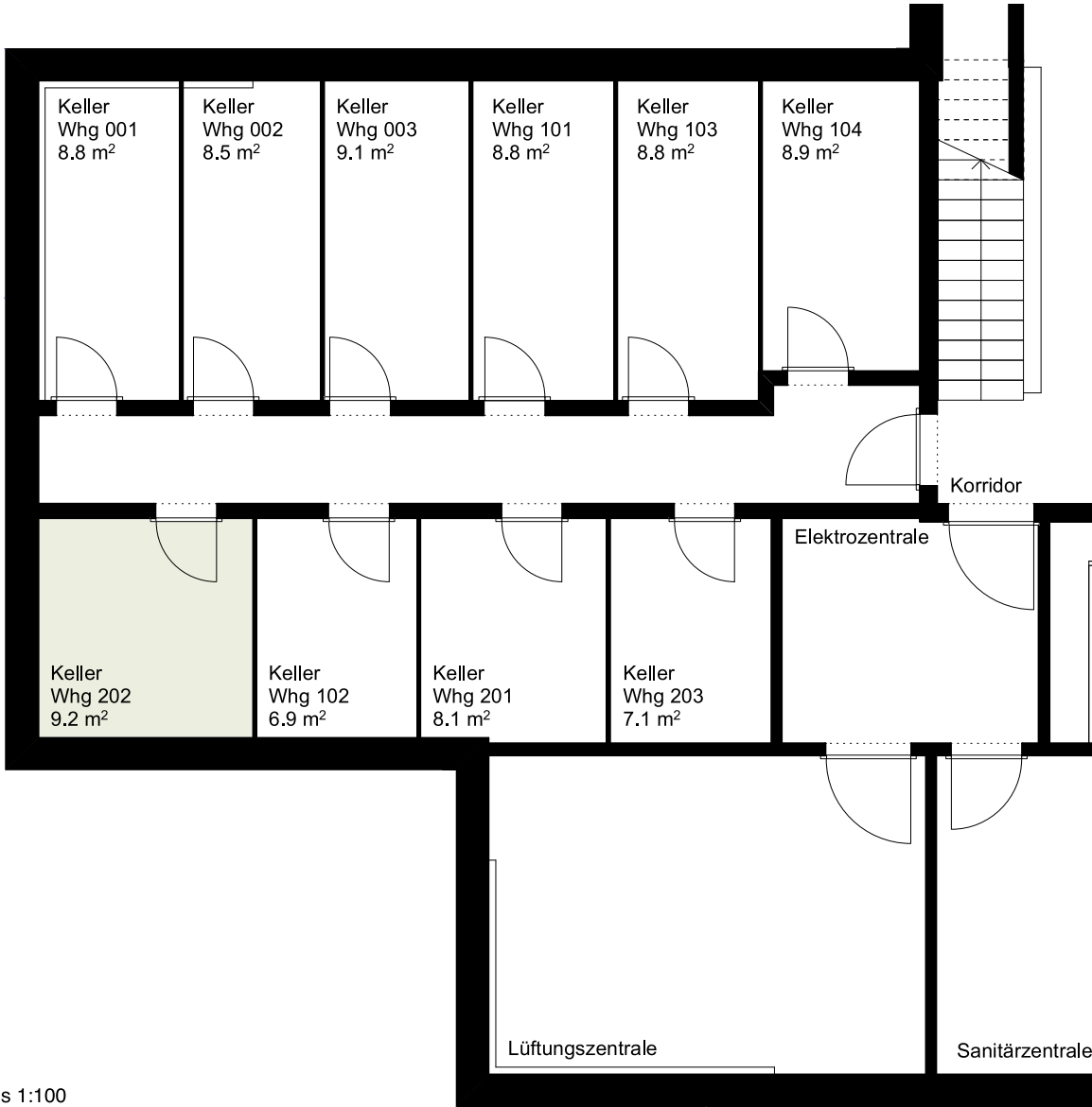
Untergeschoss 1:100
