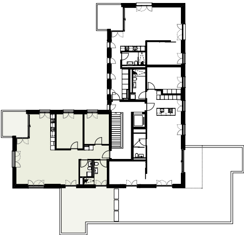
Übersicht 1:500
